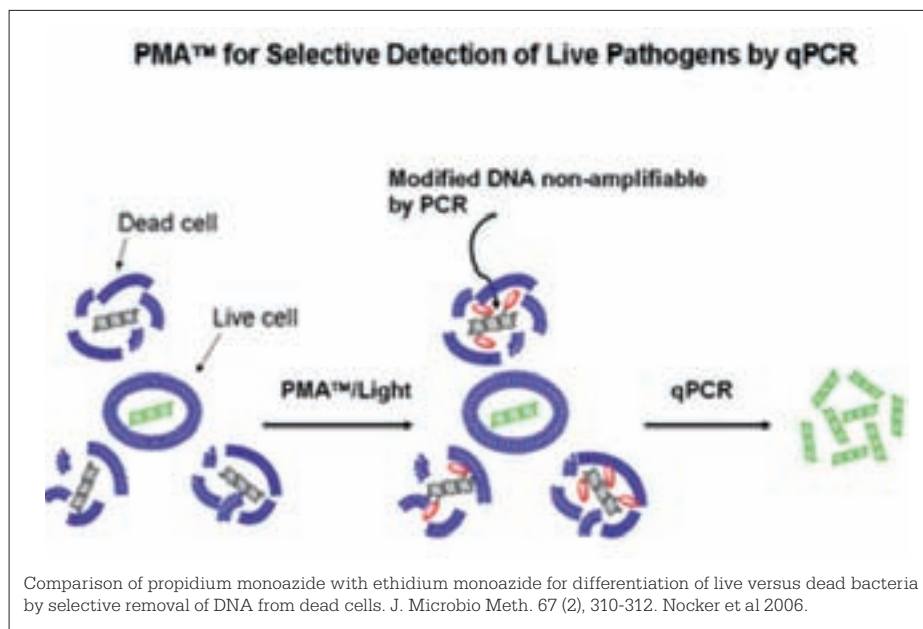
Figur 1. Propidiummonoazid (PMA) til selektiv påvisning af levende patogene bakterier med real-time PCR. PMA tilsættes prøven før PCR og binder sig til den tilgængelige DNA fra bakterier med permeable cellemembraner. Prøven belyses, og PMA-DNA bindingen bliver irreversibel, mens det overskydende ubundne PMA ændres til hydroxylamin. Efter DNA ekstraktion vil der være to DNA-fraktioner tilstede; den PMA-bundne fra døde bakterier med permeable cellemembraner, og den ubundne fra levende bakterier. Den ubundne DNA bliver denatureret og mangfoldiggjort i PCR, hvorimod den bundne DNA ikke vil være tilgængeligt for PCR-mangfoldiggørelse.
